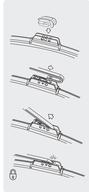
Рычаг с крючком
