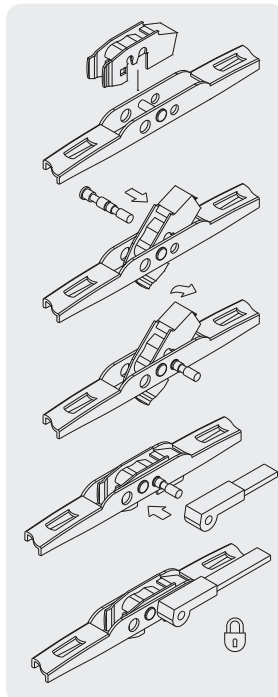
Рычаг с отверстием
