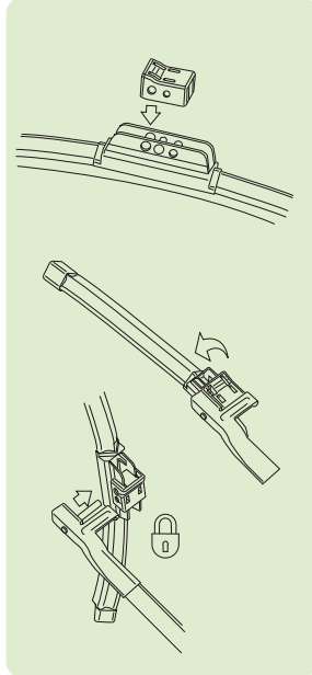
Рычаг с боковой шпилькой BOSCH type II
